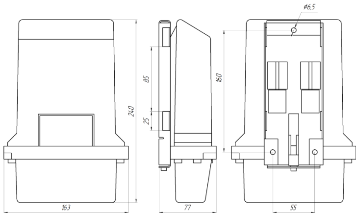
Рисунок А.1 - Размеры счетчика в исполнении С
